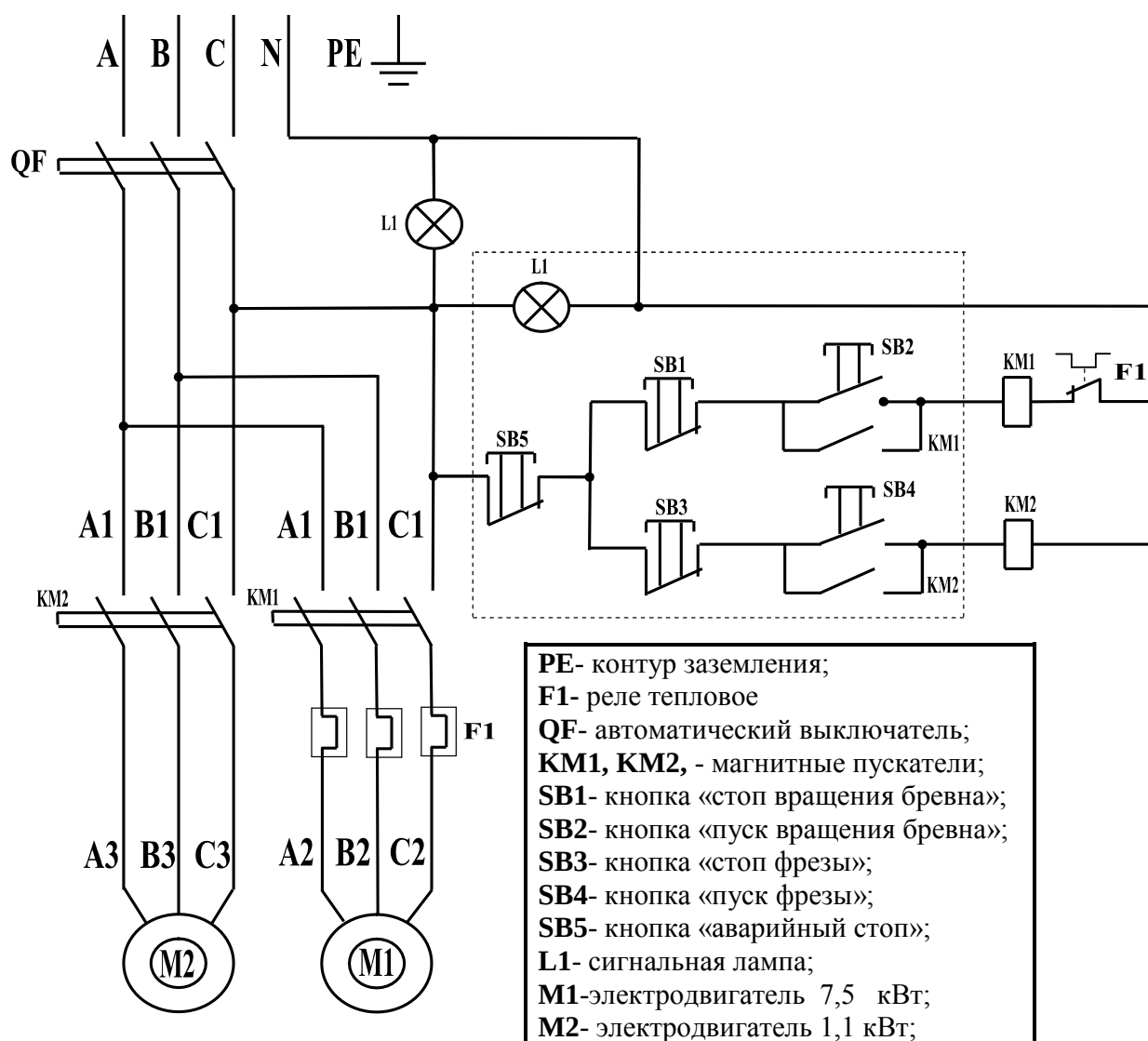
Рис. 3 Схема электрическая принципиальная
